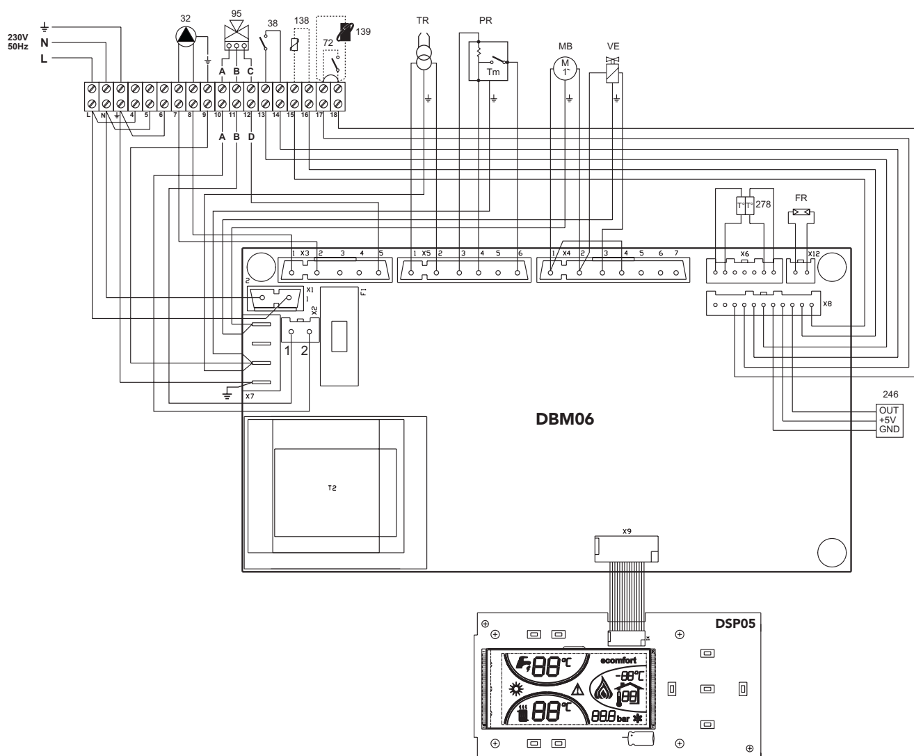
fig. 33 - Schema elettrico
