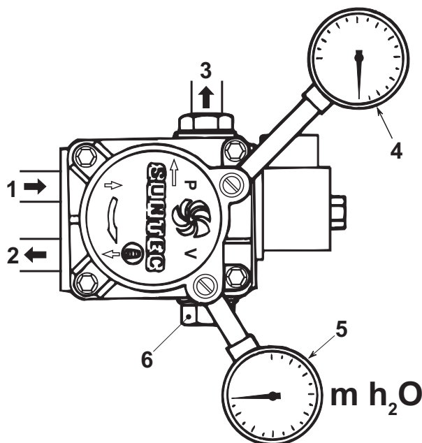
fig. 24 - Pompa
