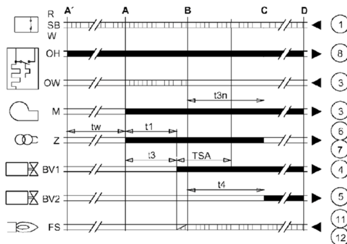
fig. 29 - Ciclo dell'apparecchiatura
