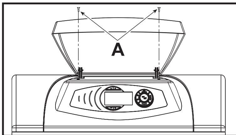
fig. 22 - Accesso alla morsettiera
