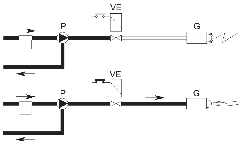
fig. 28 - Avviamento
