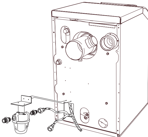
fig. 17 - Installazione filtro combustibile
