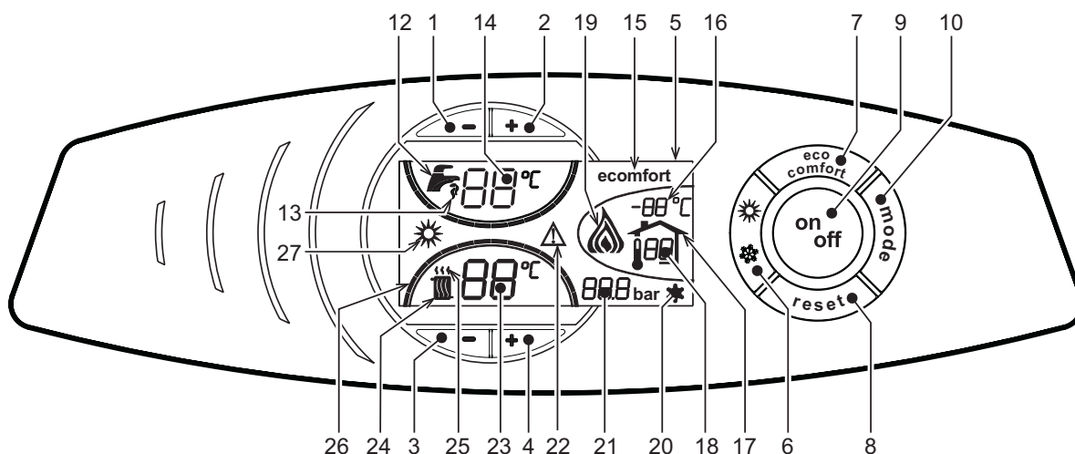
fig. 1 - Pannello di controllo
