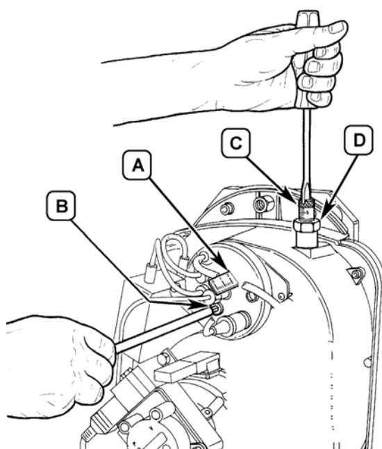
fig. 26 - Regolazione bruciatore
